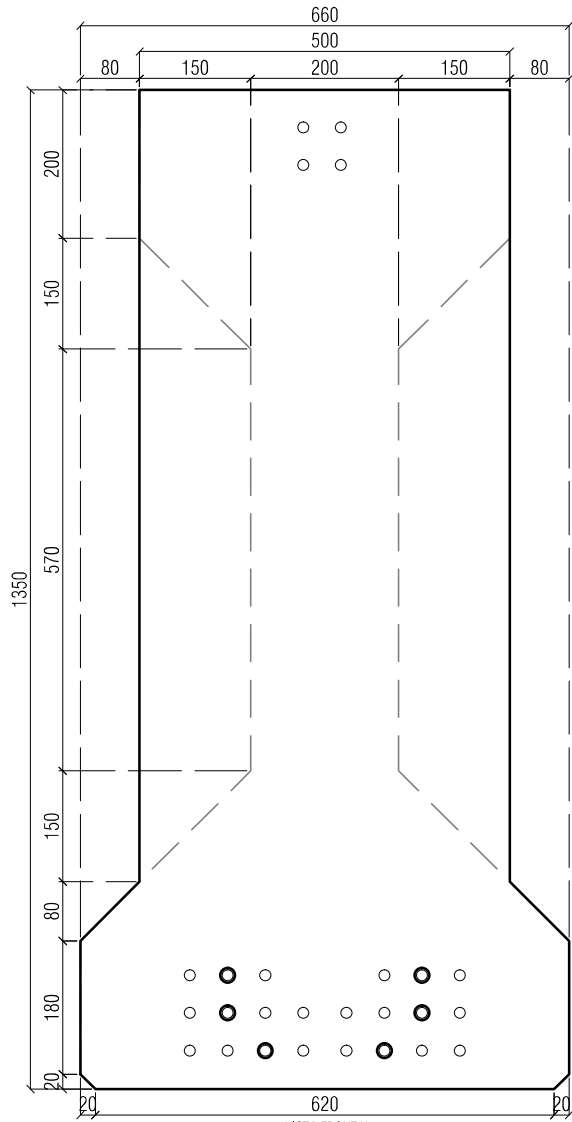
VISTA FRONTAL SECCIÓN MACIZADA Esc. 1:10
