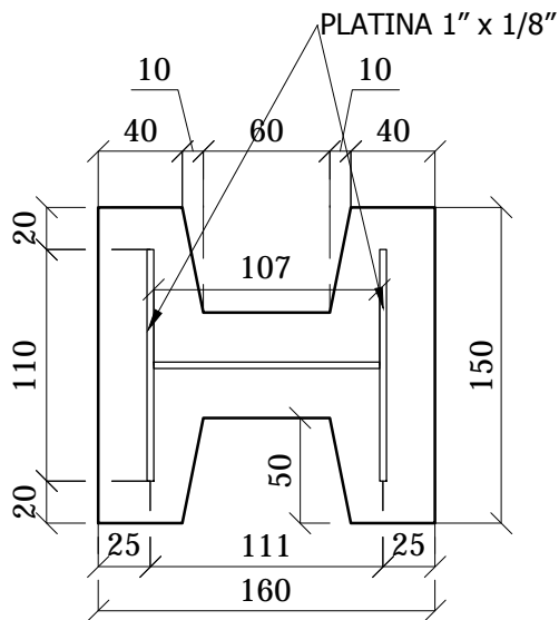
VISTA EN PLANTA Esc. 1:5
